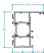
Dormant 70 sans aile
