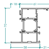
Dormant 70 avec aile
