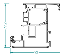
Porte-Fenêtre serrure
